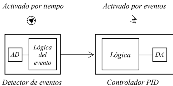
Figura 15 Control PID basado en eventos de Árzén
