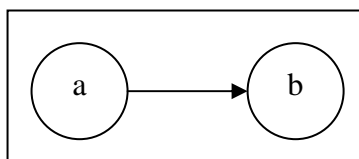
FIG. 0.1. Grafo dirigido.
