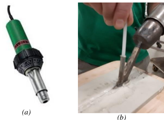
Figura 9. (a) Soprador de ar quente (Leister) e (b) Execução do processo HGW.
