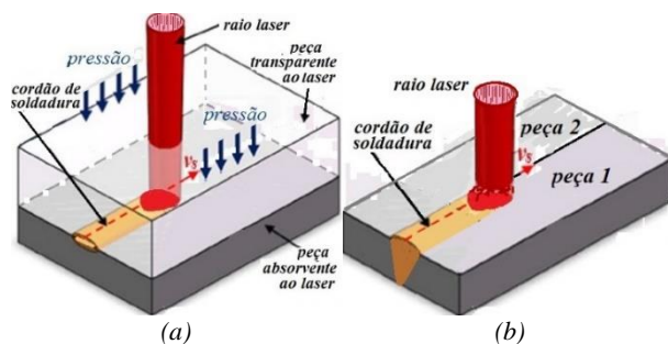
Figura 5. Princípio de soldadura laser de junta (a) sobreposta; (b) de topo. Fonte: Adaptado de [13].
