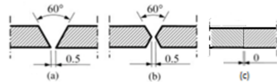
Figura 8. Esquema de preparação das juntas: (a) em V, (b) duplo V e (c) em contato total.
